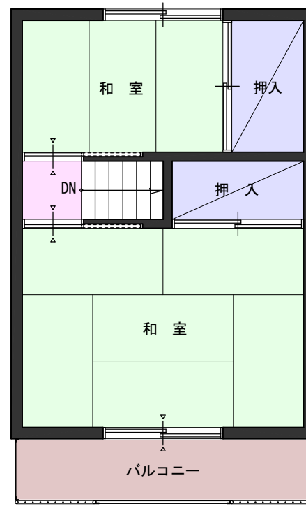
2 F
