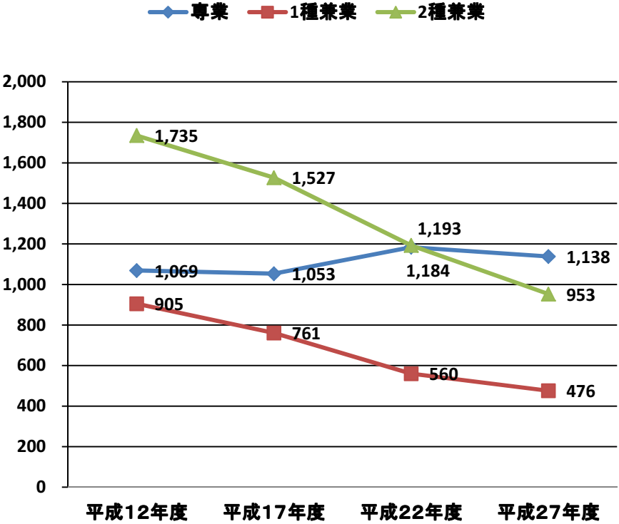
専業別割合(%)
