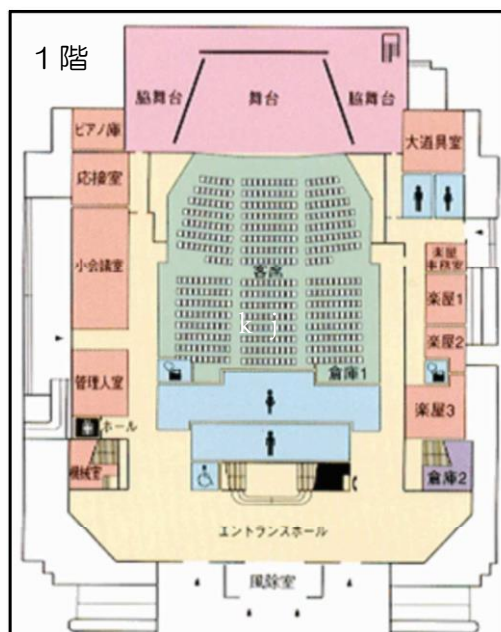
▼平面図
