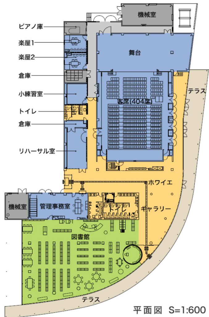
▶平面図
