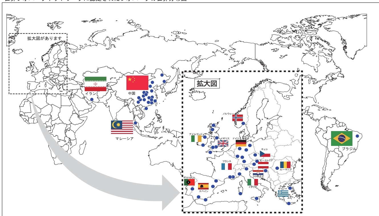
世界ジオパークネットワークに認定されたジオパークの世界分布図
