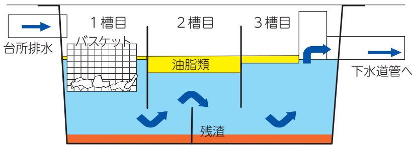
油取ますのしくみ(ますを横割した様子)
