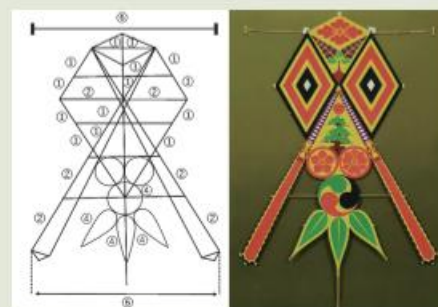
ケンボーソーの設計図 (雲仙市吾妻町ハタ保存会提供)
