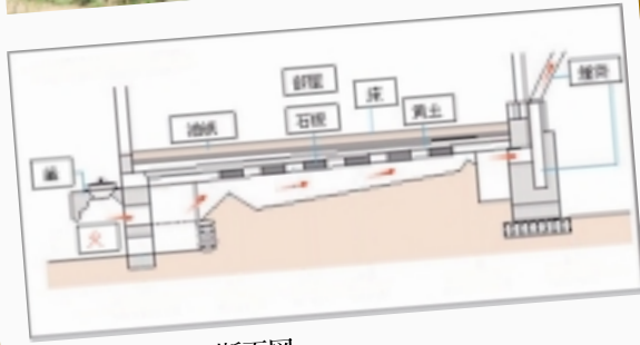
昔のオンドルの断面図
